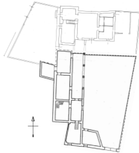
5 Pianta Piano Terra
