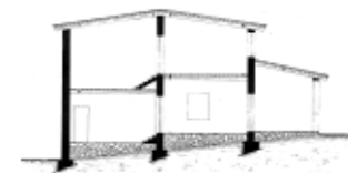
Sezione K-K
