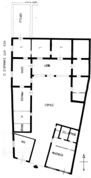
1 Pianta Piano Terra
